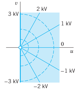
Fig. 406. Example 2: w -plane
