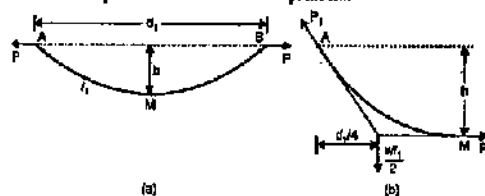
FIG. 3.23. SAG CORRECTION
