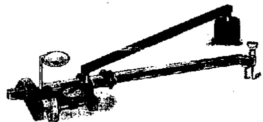
FIG. 12.11. AMSLER POLAR PLANIMETER.
