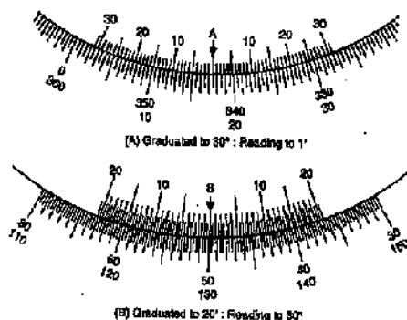
FIG. 1.11. VERNIERS TO CIRCULAR SCALES.
