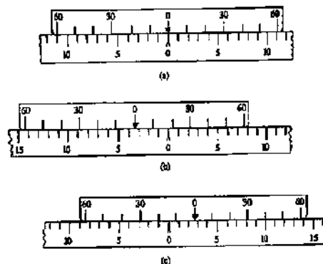
FIG. 1.9 EXTENDED VERNIER.
