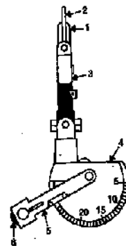
FIG. 14.7. DE LISLE'S CLINOMETER.
