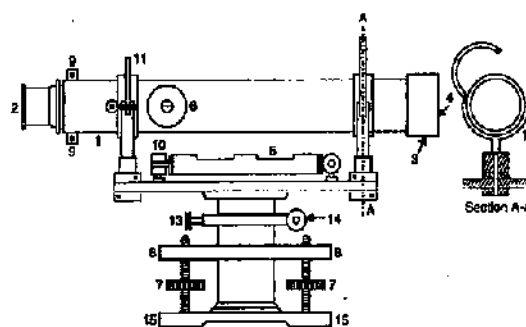
FIG. 9.7. WYE LEVEL.
