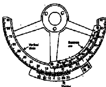
FIG. 22.26. BEAMAN STADIA ARC.
