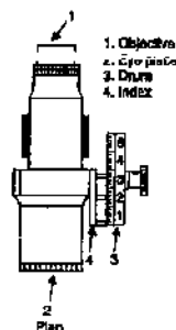
FIG. 1.12. MICROMETER MICROSCOPE.
