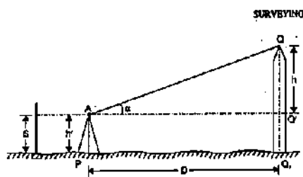
FIG. 15.1. BASE ACCESSIBLE
