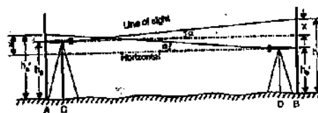
FIG. 16.3. TWO PEG TEST (METHOD A).
