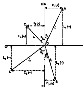
FIG. 8.1. LATITUDE AND DEPARTURE
