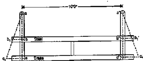
FIG. 3.36. THE COLBY APPARATUS.
