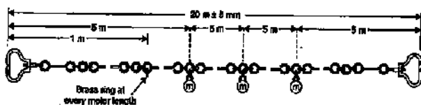
FIG. 3.4. 20-METER CHAIN
