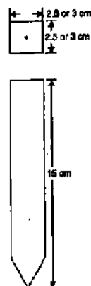
FIG. 3.16. WOODEN PEG.
