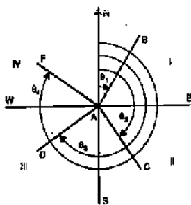
FIG. 5.1 W.C.B. SYSTEM.
