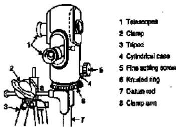
FIG. 4.19. THE SITE SQUARE.
